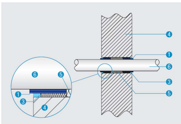
Detalle A
